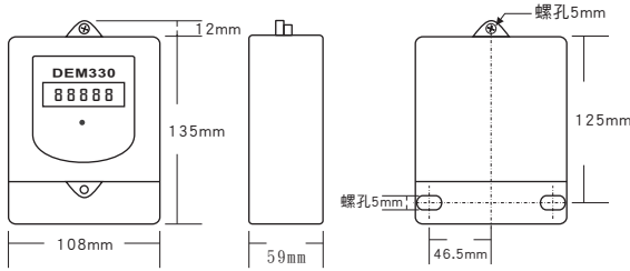
DEM330 10(30)A 單相三線電子式電度表 重量: 0.5KG
