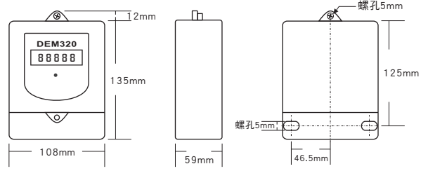
DEM320 10(30)A 單相二線電子式電度表 重量: 0.5KG
