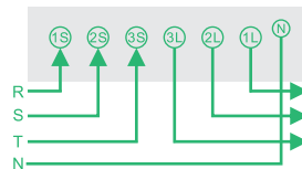
接線圖4: 三相四線 直接接入式
