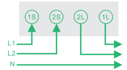
接線圖2
