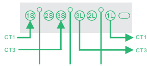
接線圖5: 三相三線 配合變比器5A
