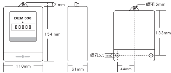
DEM530M 20(80)A 單相三線電子式電度表 重量: 0.7KG
