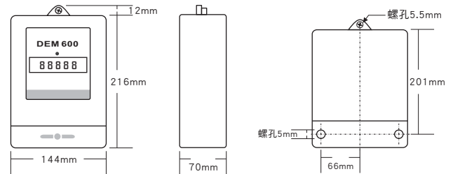
DEM600M 三相電子式電度表 重量: 1.6KG
