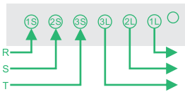
接線圖3: 三相三線 直接接入式
