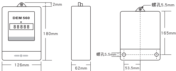
DEM560M 10(50)A 三相三線電子式電度表 重量: 1KG
