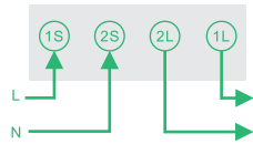
接線圖1
