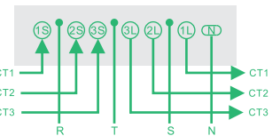
接線圖6: 三相四線 配合變比器5A
